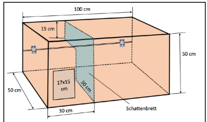
Skizze eines Schleihereulen Nistkastens
